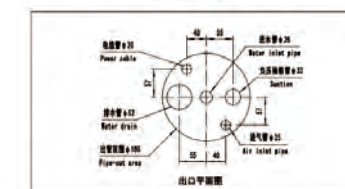
出口平面圖
